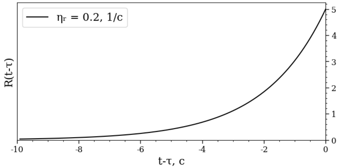
Рисунок 2.1 – Экспоненциальное ядро интегрального оператора нелокальной модели
