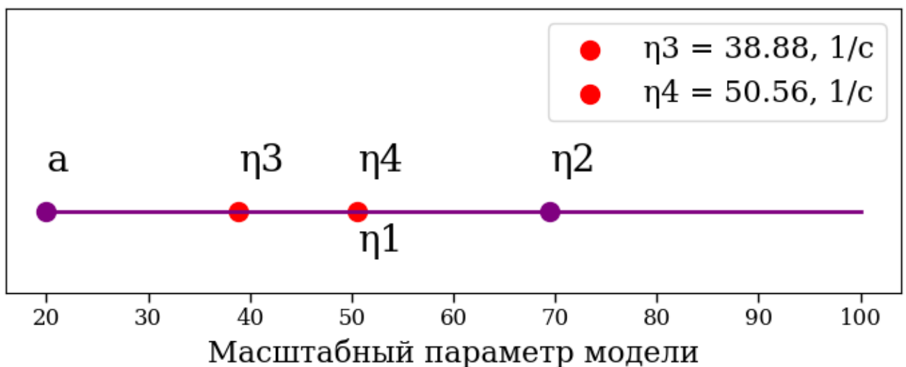
Рисунок 3.3 – График деления интервала в пропорции «золотого сечения» на второй итерации
