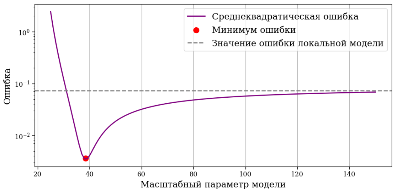
Рисунок 3.3 – График среднеквадратичной ошибки в зависимости от масштабного параметра модели полученный в результате калибровки модели
