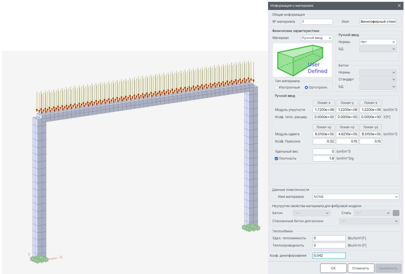
Рисунок 3.17 – Общий вид конечно-элементной модели, собранной из трехмерных твердотельных конечных элементов, построенная в расчетном комплексе MIDAS-Civil . Заданные свойства материала
