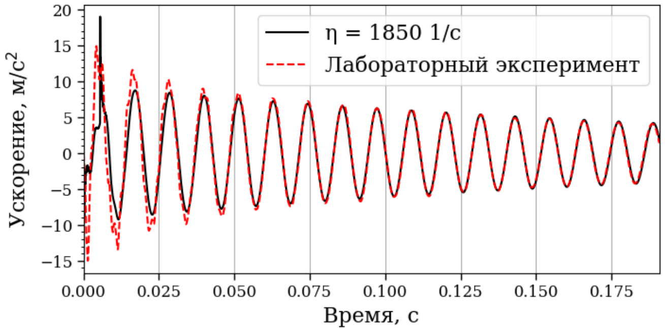
Рисунок 4.10 – Сравнение результатов для балки 1700К с результатами откалиброванной нелокальной модели, при импульсном воздействии, приложенном в середине пролёта.
