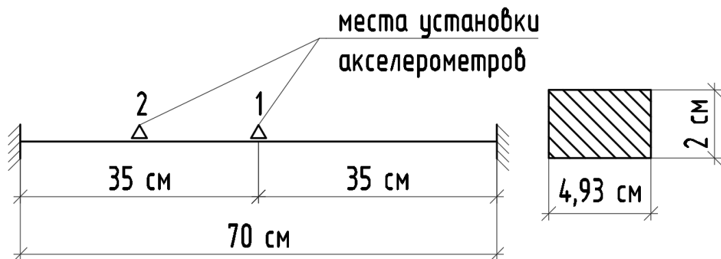
Рисунок 4.8 – Расчетная схема экспериментальной установки для жестко заземленной балки по краям
