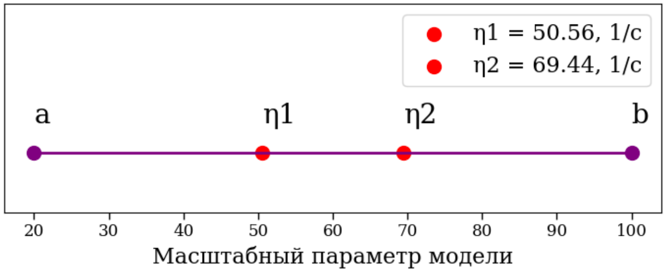
Рисунок 3.2 – Деление интервала [a, b] в пропорции «золотого сечения» на первой итерации
